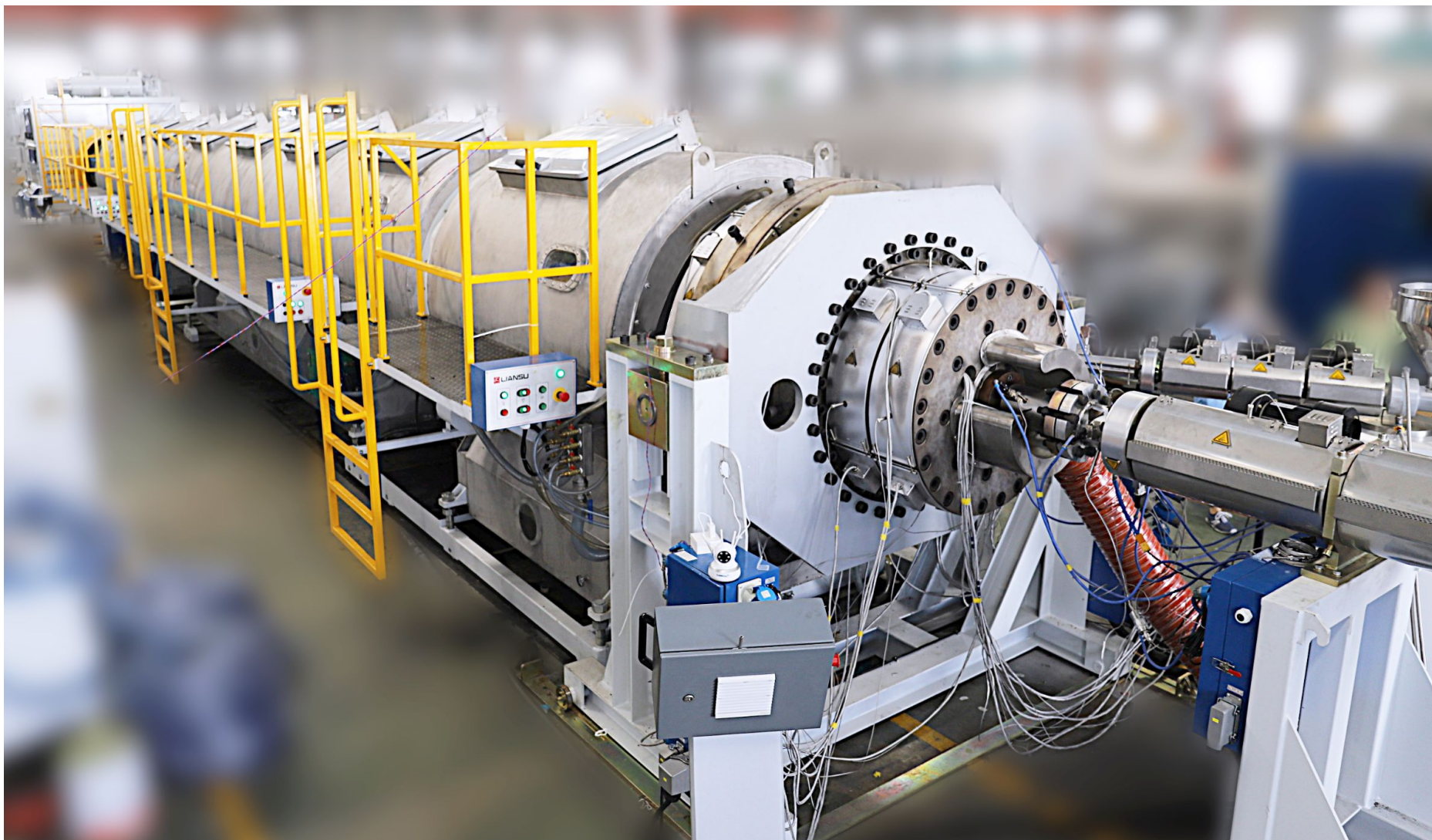
Головка оснащена системой вентиляции, что сокращает длину охлаждения
